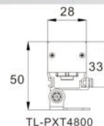
TL-PXT4800
