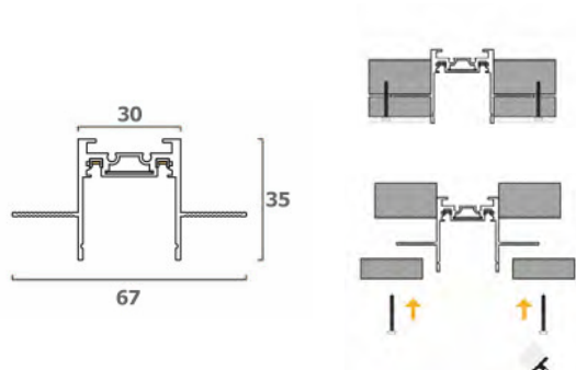
Thanh ray lắp âm
