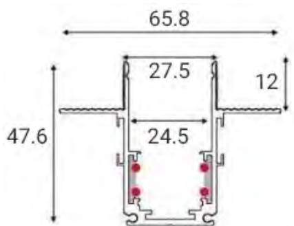
Thanh ray lắp âm
