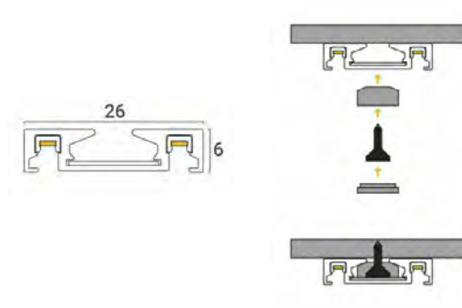
Thanh ray lắp nổi
