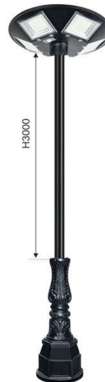
SOLAR - TRỤ 157 Ø Đèn: 550 x H125 - ABS Ø Đế: 300 x H3700 BNL: 6V - 25W - Pin : 30 AH Bóng phát sáng 300W Cảm biến ánh sáng - IP65 Thấp sáng: 8 -> 10 giờ 10.330.000đ ○●
