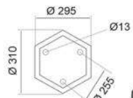
TRỤ 288 L800 x H4000 E27 x 3 14.000.000đ
