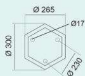
TRỤ 331 L660 x H4000 E27 x 2 9.700.000đ
