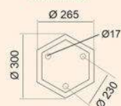
CHÂN ĐẾ 03 H630 - Nhôm 3.730.000d
