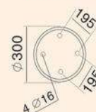
CHÂN ĐẾ 05 H1000 - Nhôm 3.780.000d
