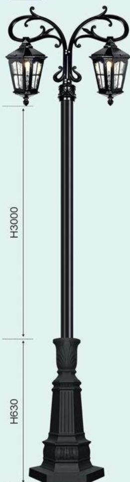
TRỤ 331 L660 x H4000 E27 x 2 9.700.000đ
