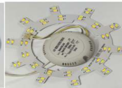
LV 7925 Ø240 18w LED 3 Màu Giá 185.000đ
