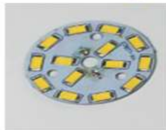
LV 1164 Ø35 LED 5W 3000K Giá 15.000đ
